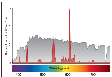
Typisches Lichtspektrum einer Energiesparlampe (Kompaktleuchtstofflampe)
